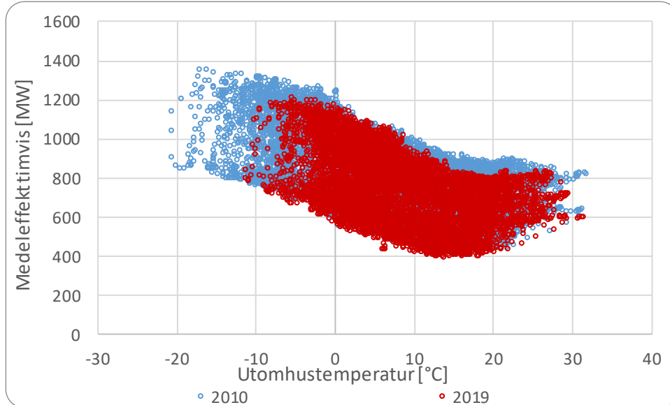
Figur 2.17-1: Timvis medeleffekt som funktion av utomhustemperatur.
