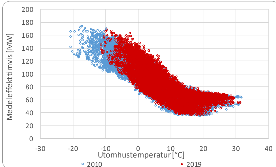
Figur 2.4-1: Timvis medeleffekt som funktion av utomhustemperatur.
