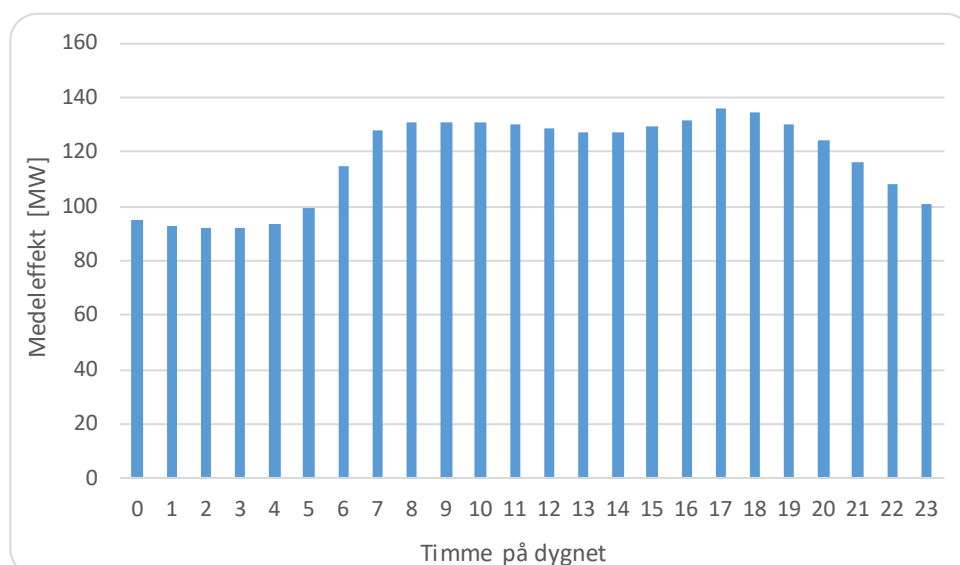
Figur 2.6-4: Medeleffekt för respektive timme på dygnet, på vardagar under vintermånaderna januari, februari, mars, november och december under år 2019.
