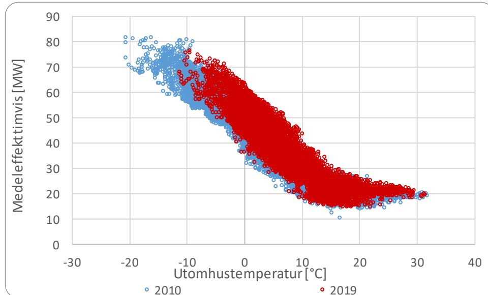
Figur 2.5-1: Timvis medeleffekt som funktion av utomhustemperatur.
