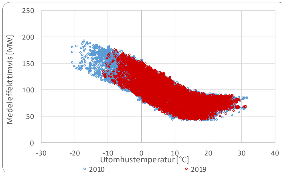
Figur 2.6-1: Timvis medeleffekt som funktion av utomhustemperatur.
