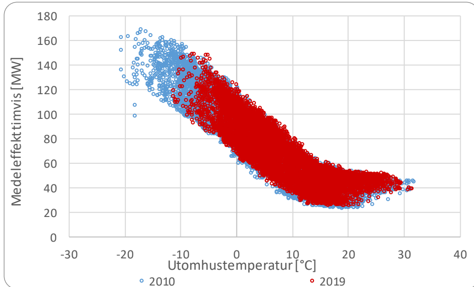
Figur 2.18-1: Timvis medeleffekt som funktion av utomhustemperatur.
