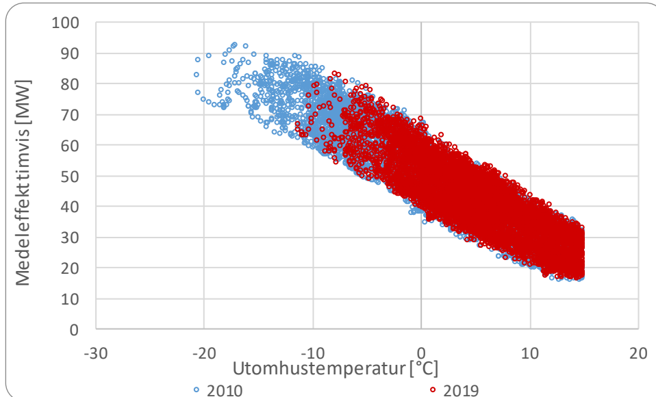
Figur 2.3-1: Timvis medeleffekt som funktion av utomhustemperatur.
