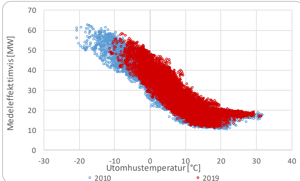
Figur 2.11-1: Timvis medeleffekt som funktion av utomhustemperatur.
