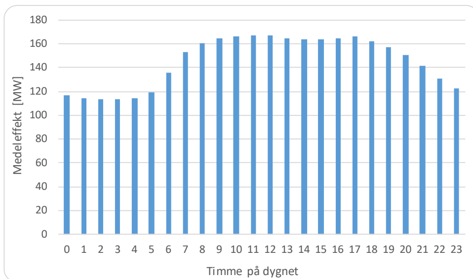
Figur 2.7-5: Medeleffekt för respektive timme på dygnet, på vardagar under vintermånaderna januari, februari, mars, november och december under år 2019.
