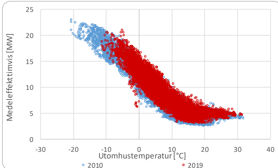
Figur 2.8-1: Timvis medeleffekt som funktion av utomhustemperatur.
