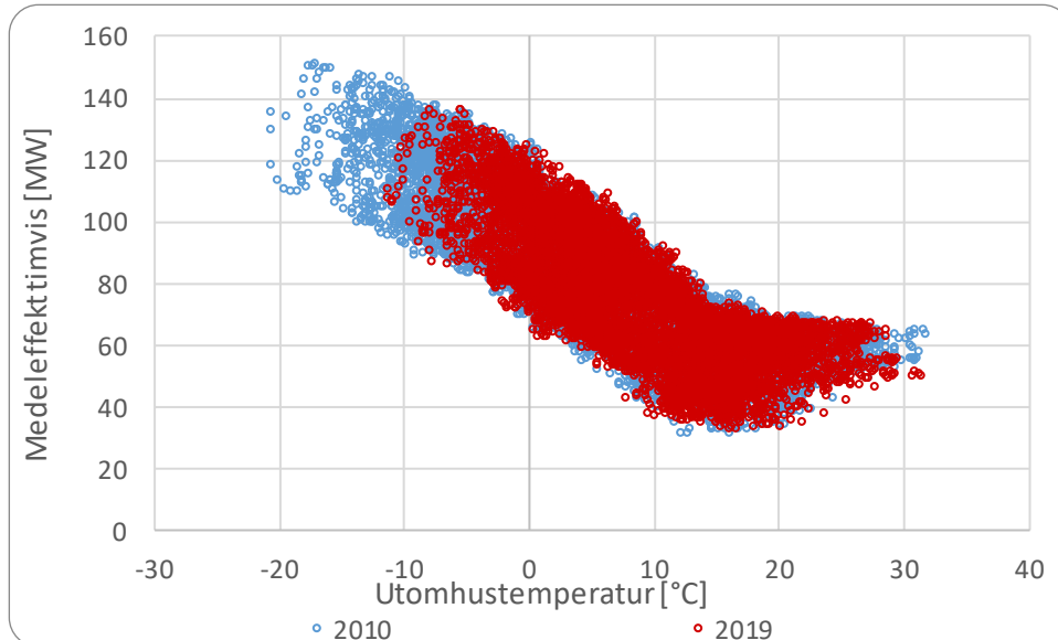
Figur 2.19-1: Timvis medeleffekt som funktion av utomhustemperatur.
