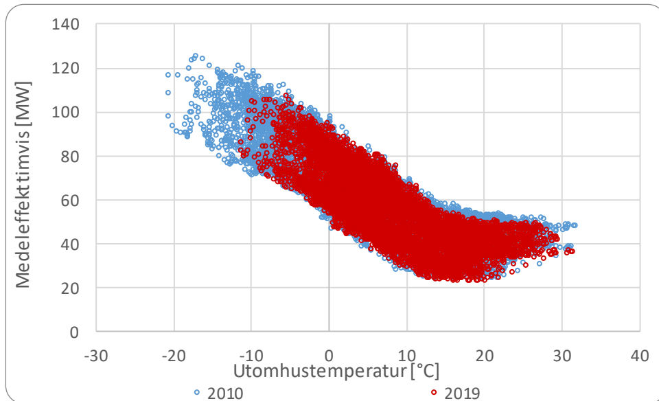
Figur 2.16-1: Timvis medeleffekt som funktion av utomhustemperatur.
