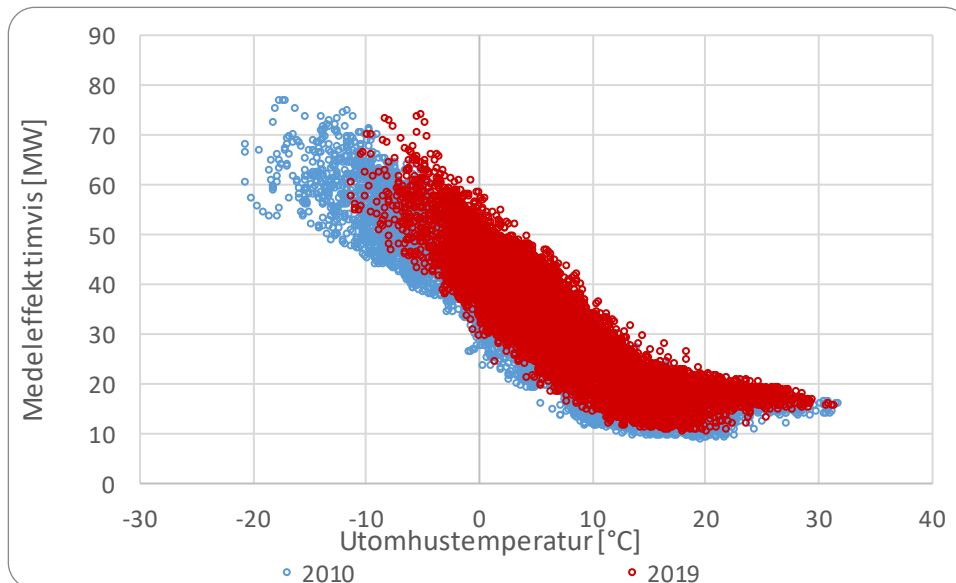
Figur 2.21-1: Timvis medeleffekt som funktion av utomhustemperatur.
