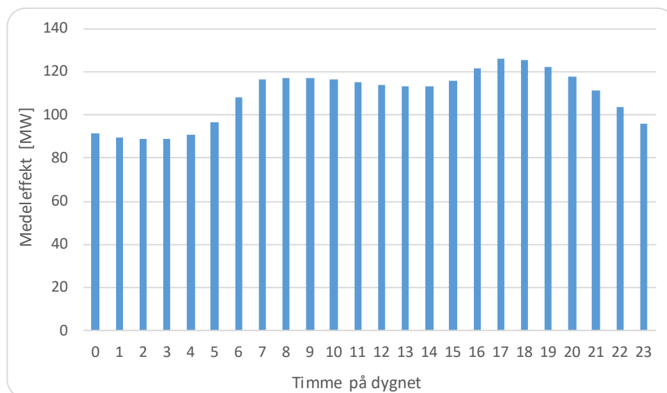
Figur 2.4-4: Medeleffekt för respektive timme på dygnet, på vardagar under vintermånaderna januari, februari, mars, november och december under år 2019.
