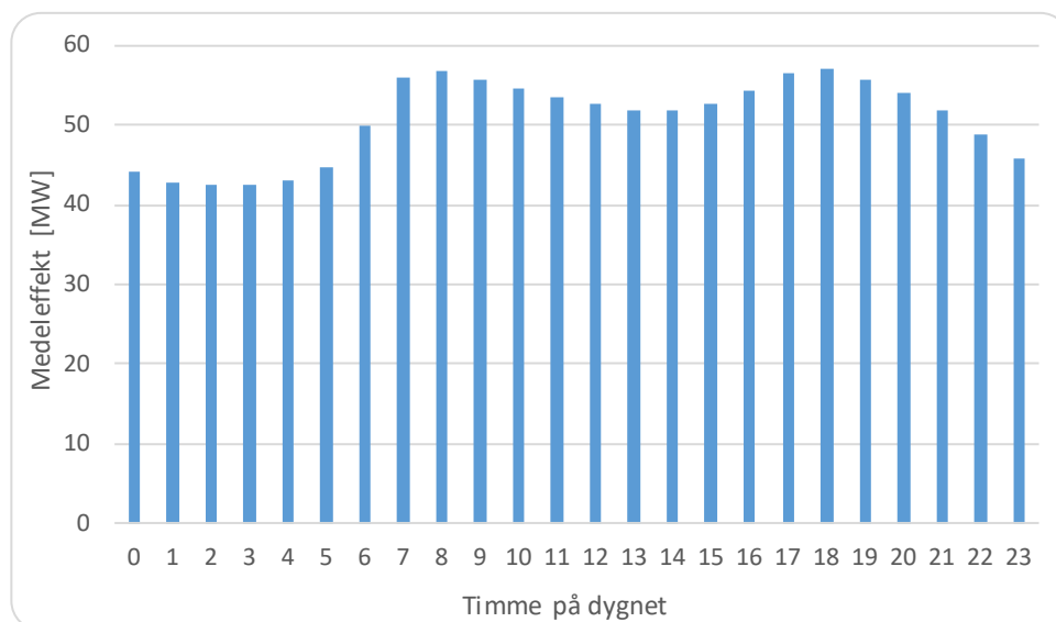
Figur 2.3-4: Medeleffekt för respektive timme på dygnet, på vardagar under vintermånaderna januari, februari, mars, november och december under år 2019.
