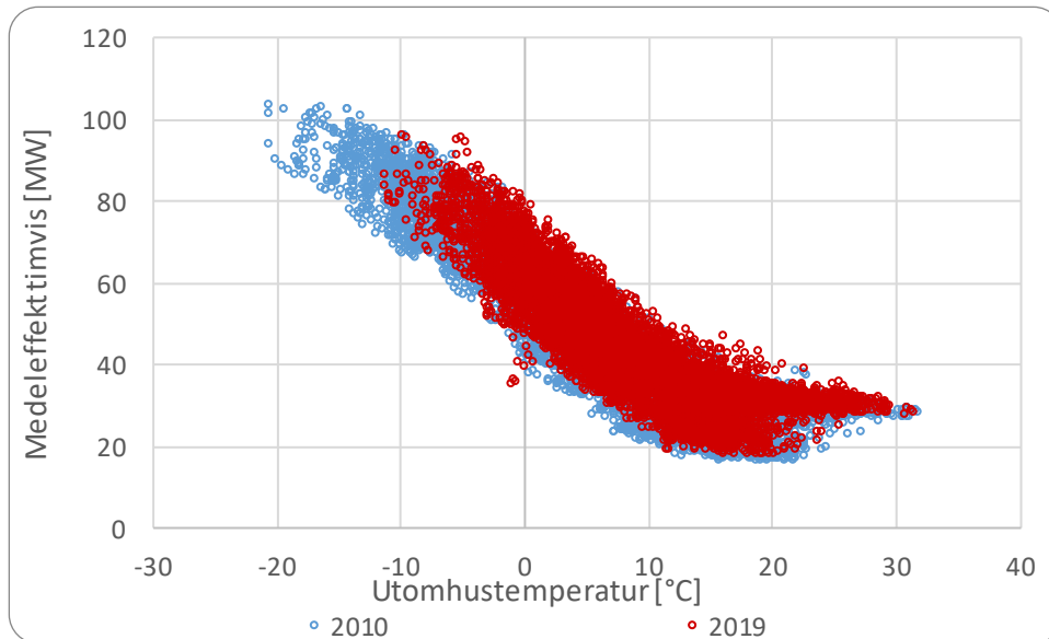
Figur 2.22-1: Timvis medeleffekt som funktion av utomhustemperatur.
