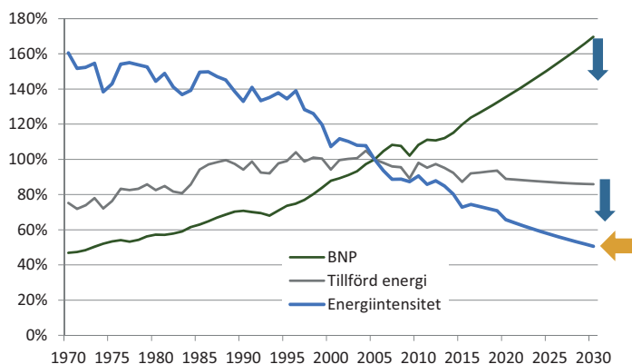
Referensfallets energiintensitetsutveckling, 2005 – 2030.
