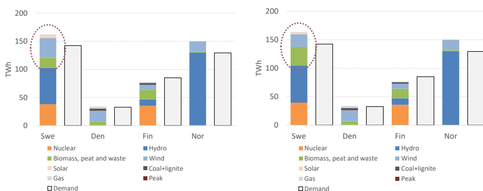
Figur 1: Den beräknade elproduktionen år 2030 (med EPOD-modellen) i de fyra nordiska länderna i "RESvind" (till vänster) respektive "RESbio" (till höger).
