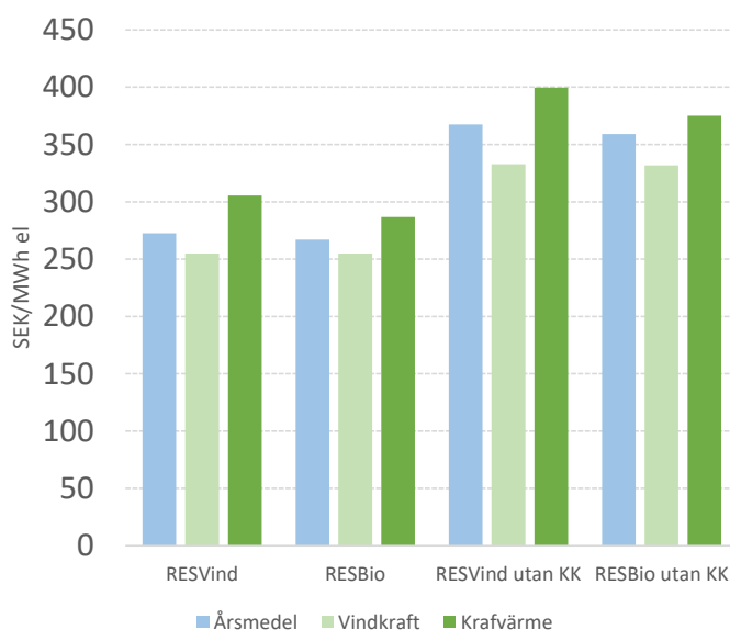
Figur 11: Genomsnittligt årsmedelelpris och produktionsprofilvägda årsmedelelpriser för vindkraft och kraftvärme.
